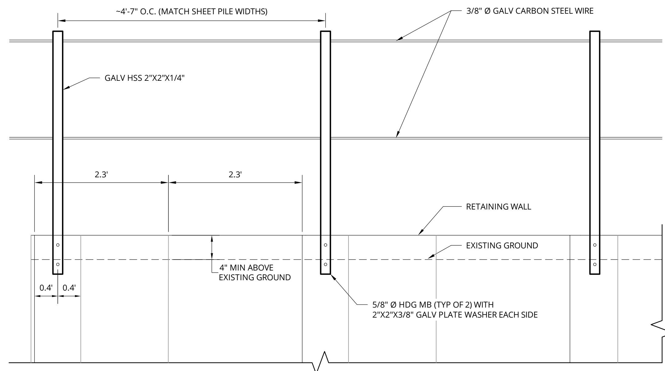
ELEVATION
